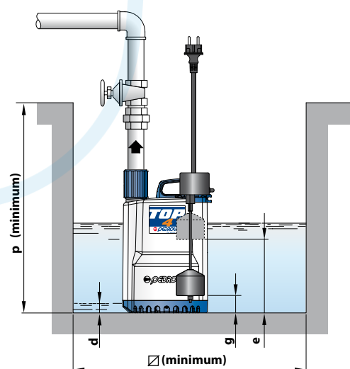
Installation typique
