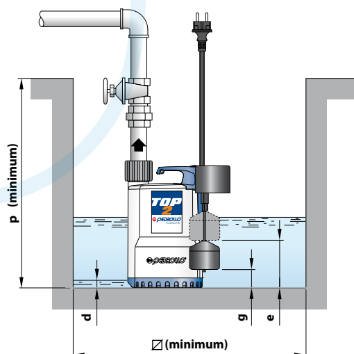
Installation typique
