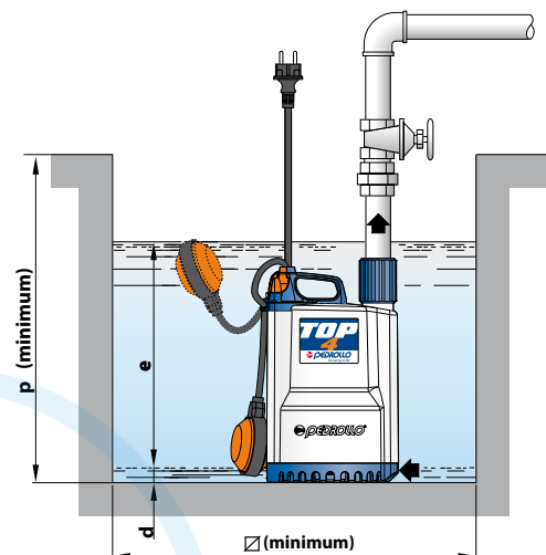
Installation typique
