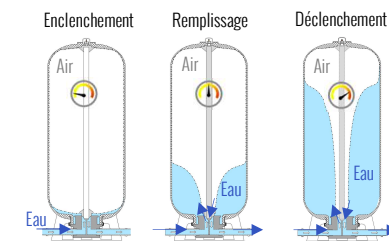
Cycle de pression des réservoirs à vessie Compose It™
