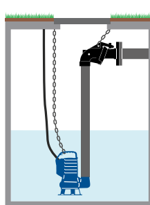
AVEC DISPOSITIF D'ACCOUPLEMENT EXTERNE
