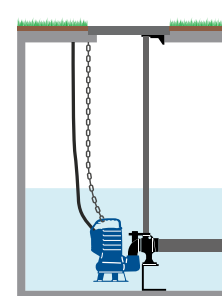
AVEC DISPOSITIF D'ACCOUPLEMENT AU FOND
