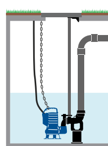
AVEC DISPOSITIF D'ACCOUPLEMENT AU FOND
