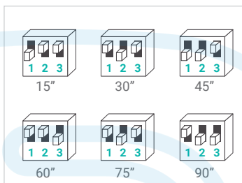
Fonction fluxostat (tempo d'amorçage)
