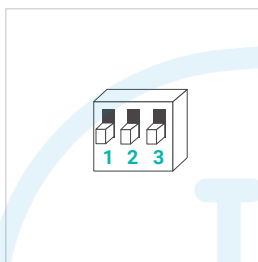
Fonction remplissage (citerne)
