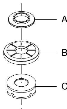
Fig. 7 Bague d'arrêt (parties mobile et fixe) et cône de serrage
