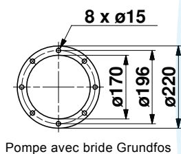
Pompe avec bride Grundfos
