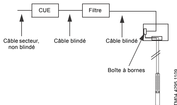
Fig. 23 Exemple d'installation sur sites sensibles aux interférences CEM
